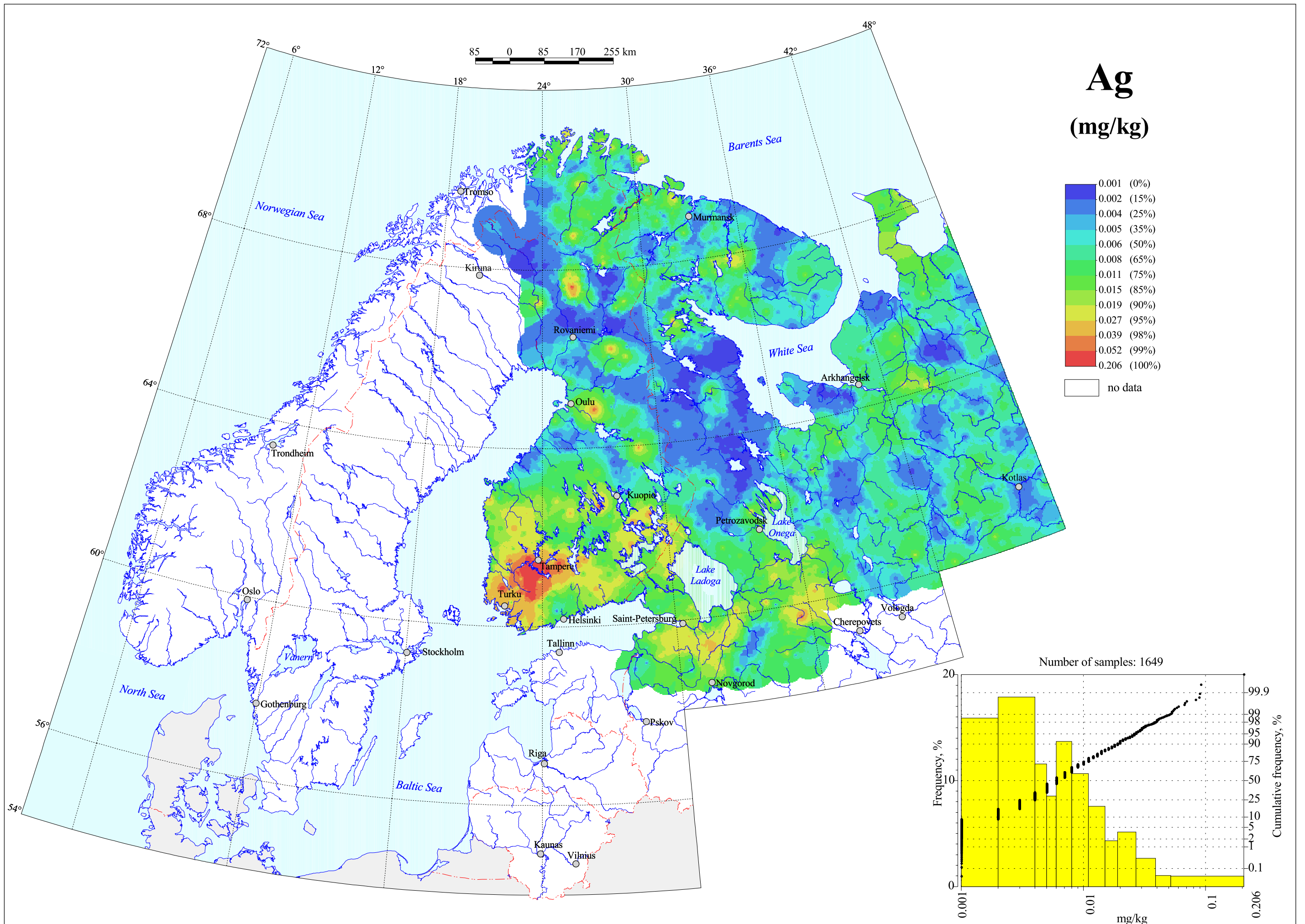
Silver in C-horizon, Grain Size <2 mm, Aqua regia Extraction
